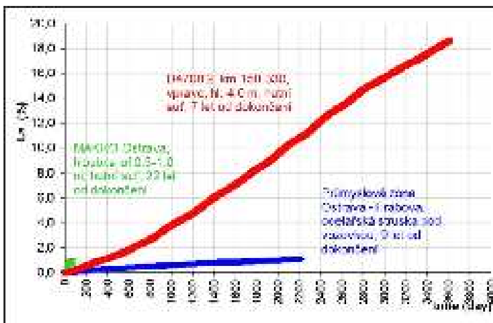
Obr. P5.5: Průběh přírůstu vertikální deformace (lineárního bobtnání) vzorků studeného odvalu v čase za normálních podmínek
