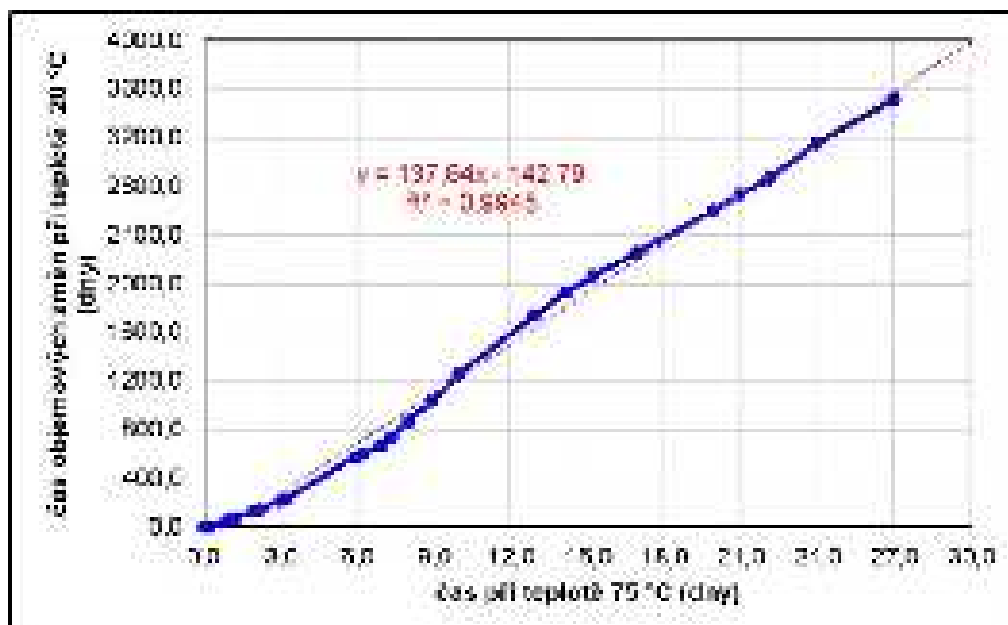
Obr. P5.6: Korelace mezi vývojem lineárního bobtnání při 75 °C a za standardních podmínek (dálnice D47, km 150,330, hloubka 4,0 m)
