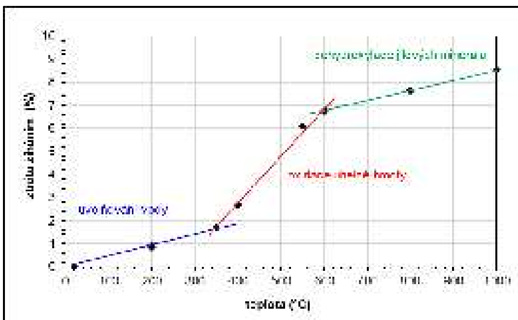
Obr. P4.2: Ztráta žháním po 2 hodinách při dané teplotě v oxidační atmosféře. Příklad jílovce s uhlými laminami (druh kořenové půdy) z podložní sloje s asociací fylosilikátů: illit 2M1, muskovit 1M, Fe-Mg chlorit
