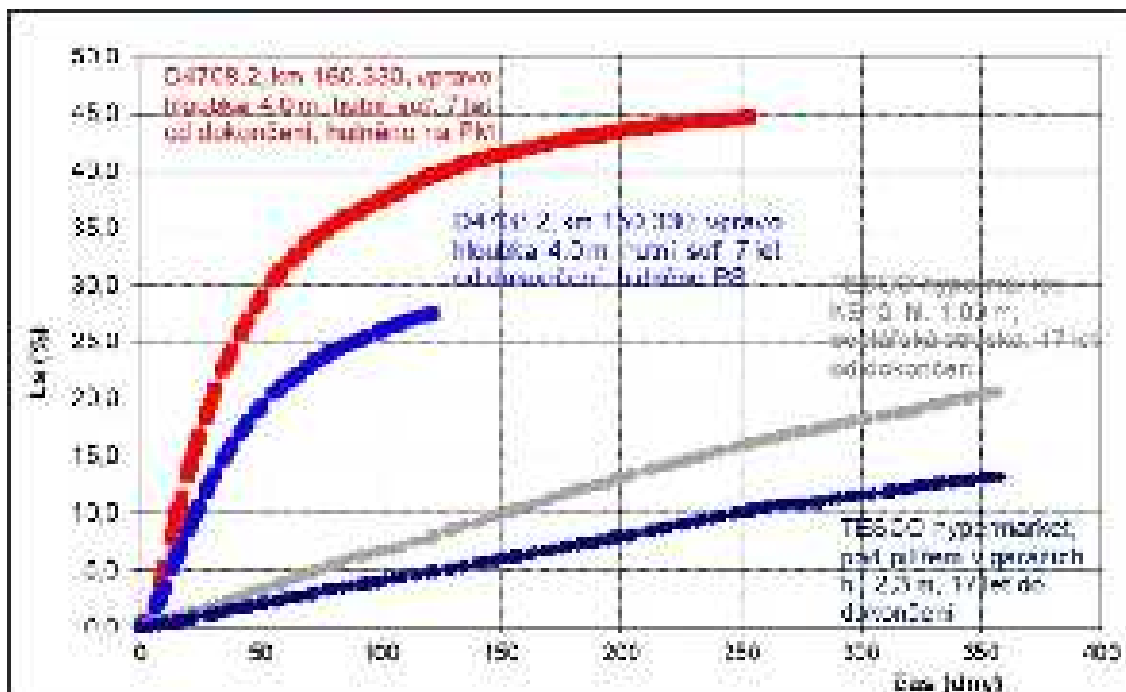
Obr. P5.3: Časový průběh přírůstu vertikální deformace (bobtnání) vzorků ocelářské strusky a studeného odvalu (hutní suť) po saturaci vodou při teplotě 75 °C
