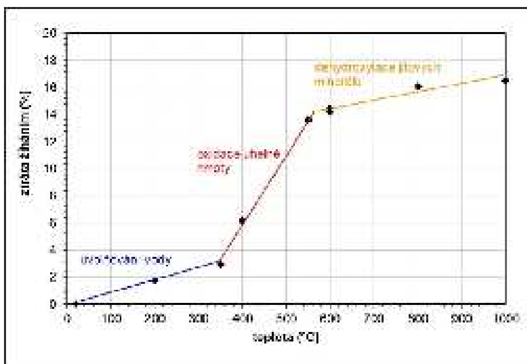
Obr.P4.1: Příklady stanovení ztrát žháním po 2 hodinách v oxidační atmosféře a stanovení ztrát žháním odpovídajících oxidaci uhelné hmototy nebo dehydroxylaci jílových minerálů a slíd v karbonských horninách (neprohořelá uhelná hlušina) – prachovce s rozptýlenou uhelnou hmotou s asociací illitu-muskovitu.
