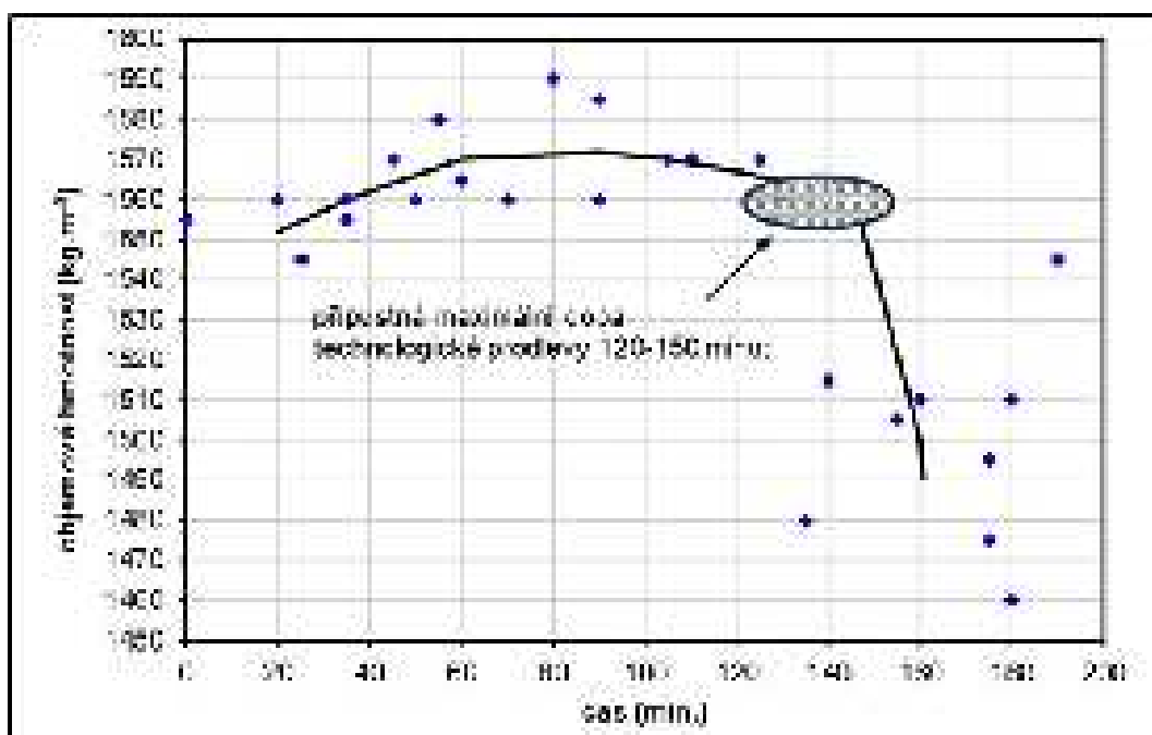
Obrázek P3.1: Příklad stanovení doby technologické prodlevy
