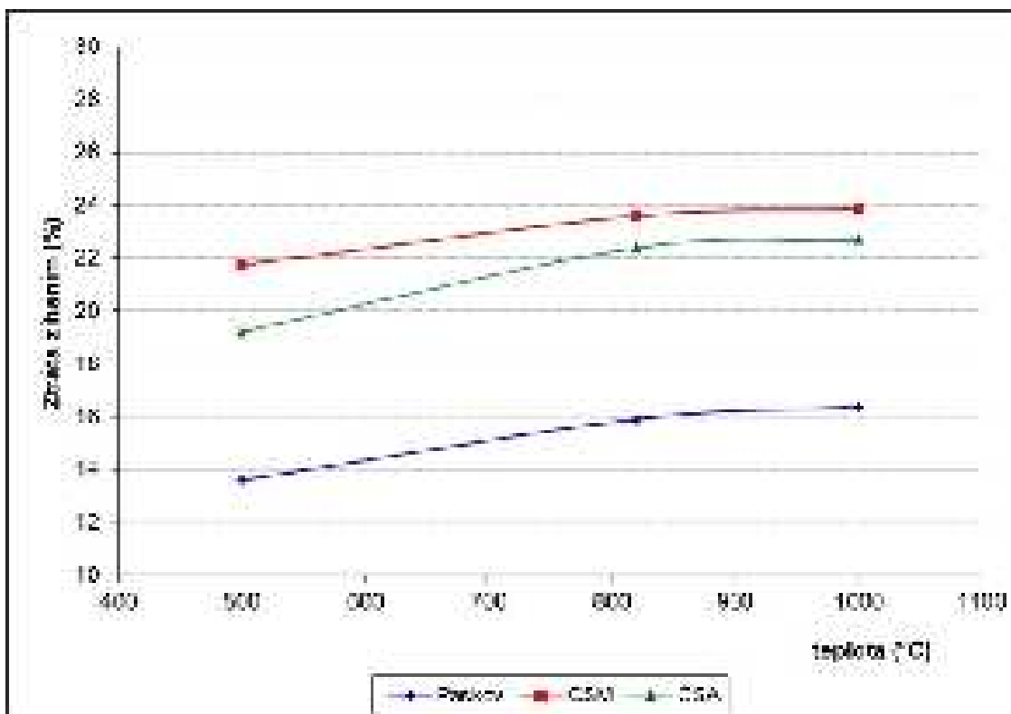
Obr. P4.4: Mediány souboru hodnot ztrát žiháním při teplotách 500 °C, 820 °C a 1000 °C pro vzorky uhelné hlušiny z úpraven Dolu ČSA, Dolu ČSM a Dolu Paskov
